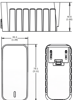
Alle Abmessungen in Millimeter (Inch), Abweichungen ± 0,5 (0.02)
