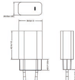
Alle Abmessungen in Millimeter (Inch), Abweichungen ± 0,5 (0.02)
