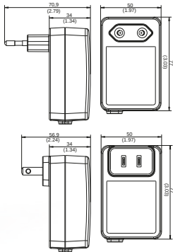
Alle Abmessungen in Millimeter (Inch), Abweichungen ± 0,5 (0,02)
