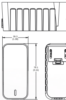
Alle Abmessungen in Millimeter (Inch), Abweichungen ± 0,5 (0.02)
