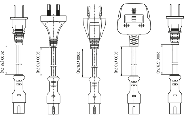
Alle Abmessungen in Millimeter (Inch), Abweichung ± 0,5 (0,02)
