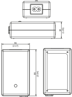
Alle Abmessungen in Millimeter (Inch), Abweichungen ± 0.5 (0.02)
