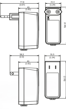
Alle Abmessungen in Millimeter (Inch), Abweichungen ± 0,5 (0,02)
