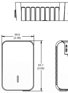
Alle Abmessungen in Millimeter (Inch), Abweichungen ± 0,5 (0.02)
