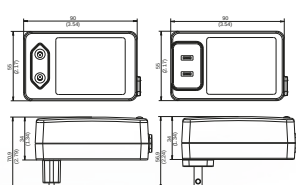
Alle Abmessungen in Millimeter (Inch), Abweichungen ± 0,5 (0.02)
