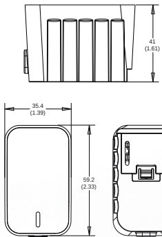
Alle Abmessungen in Millimeter (Inch), Abweichungen ± 0,5 (0.02)
