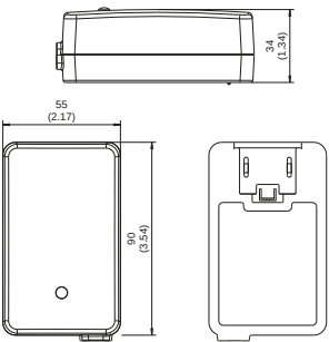
Alle Abmessungen in Millimeter (Inch), Abweichungen ± 0,5 (0,02)
