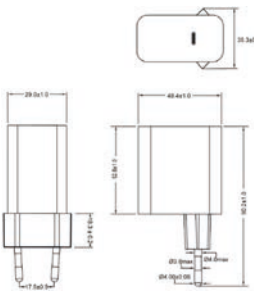
Alle Abmessungen in Millimeter (Inch), Abweichungen ± 0,5 (0.02)
