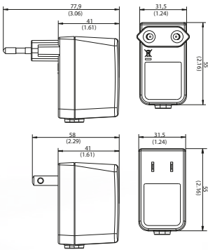
Alle Abmessungen in Millimeter (Inch), Abweichungen ± 0,5 (0,02)
