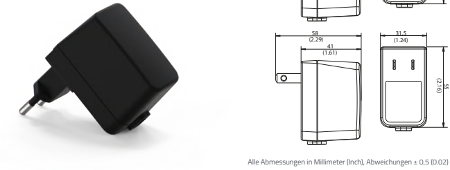
Alle Abmessungen in Millimeter (Inch), Abweichungen ± 0,5 (0,02)
