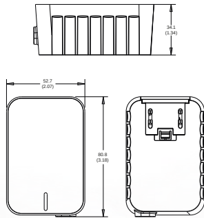
Alle Abmessungen in Millimeter (Inch), Abweichungen ± 0,5 (0.02)
