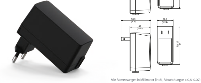
Alle Abmessungen in Millimeter (Inch), Abweichungen ± 0,5 (0,02)
