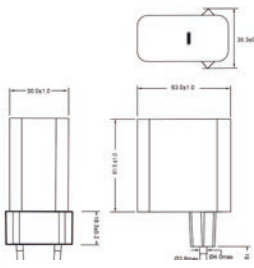
Alle Abmessungen in Millimeter (Inch), Abweichungen ± 0,5 (0.02)
