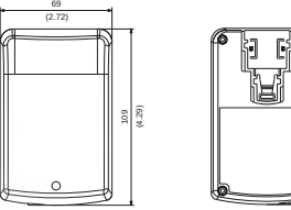
Alle Abmessungen in Millimeter (Inch), Abweichungen ± 0,5 (0.02)
