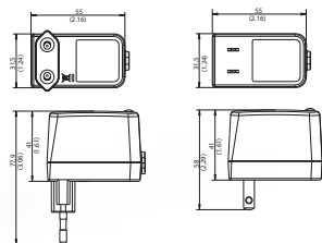
Alle Abmessungen in Millimeter (Inch), Abweichungen ± 0,5 (0.02)
