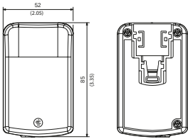
Alle Abmessungen in Millimeter (Inch), Abweichungen ± 0,5 (0.02)
