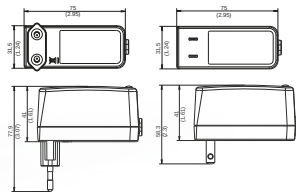
Alle Abmessungen in Millimeter (Inch), Abweichungen ± 0,5 (0.02)
